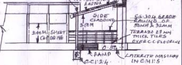
SECTION M-N.
